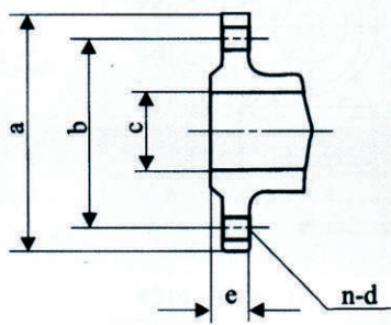
进口法兰
