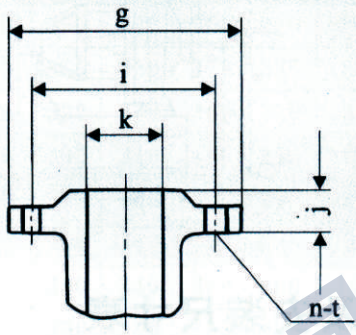
出口法兰
